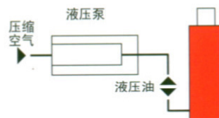
典型配置 单作用油缸配置图
